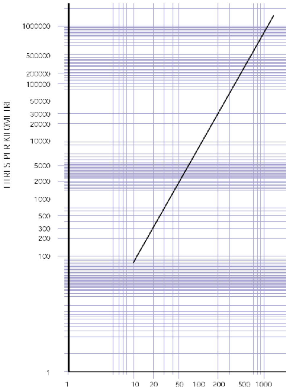
Рисунок 29. Количество воды, необходимое для заполнения 1 км трубопровода, для проведения испытаний под давлением.
