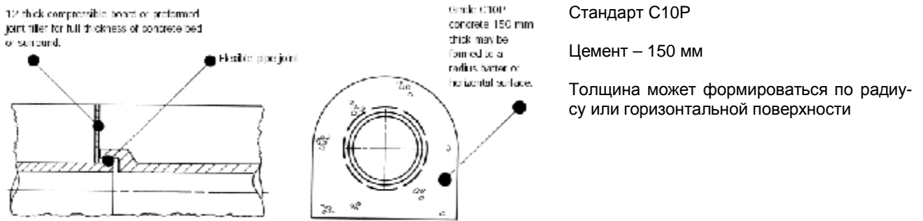
Рисунок 23. Целесообразный способ бетонирования трубы.
