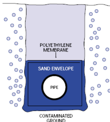
Рисунок 24. Вид траншеи в условиях зараженной местности.
