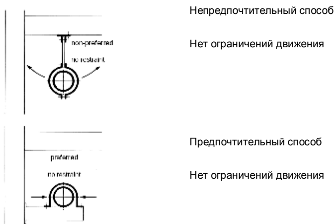
Рисунок 27. Предпочтительный наземный способ крепления
