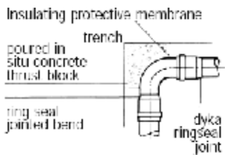
Упор при изгибе 90°
