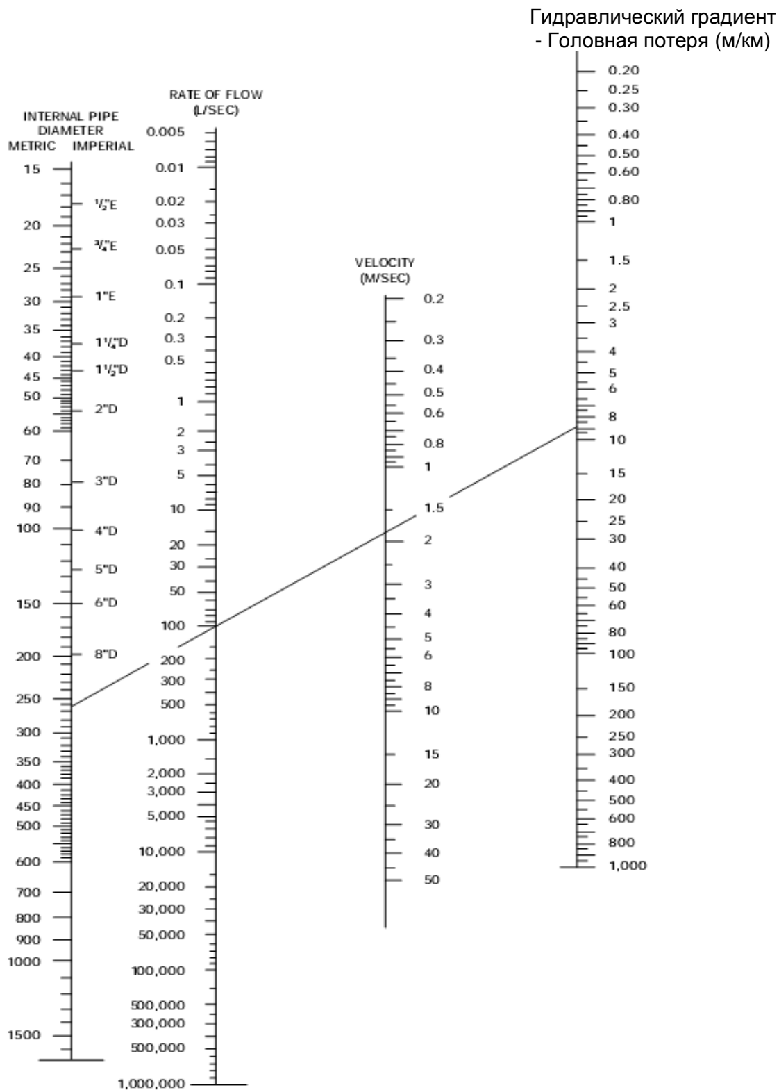
Рисунок 11 Расчетный график головной потери
